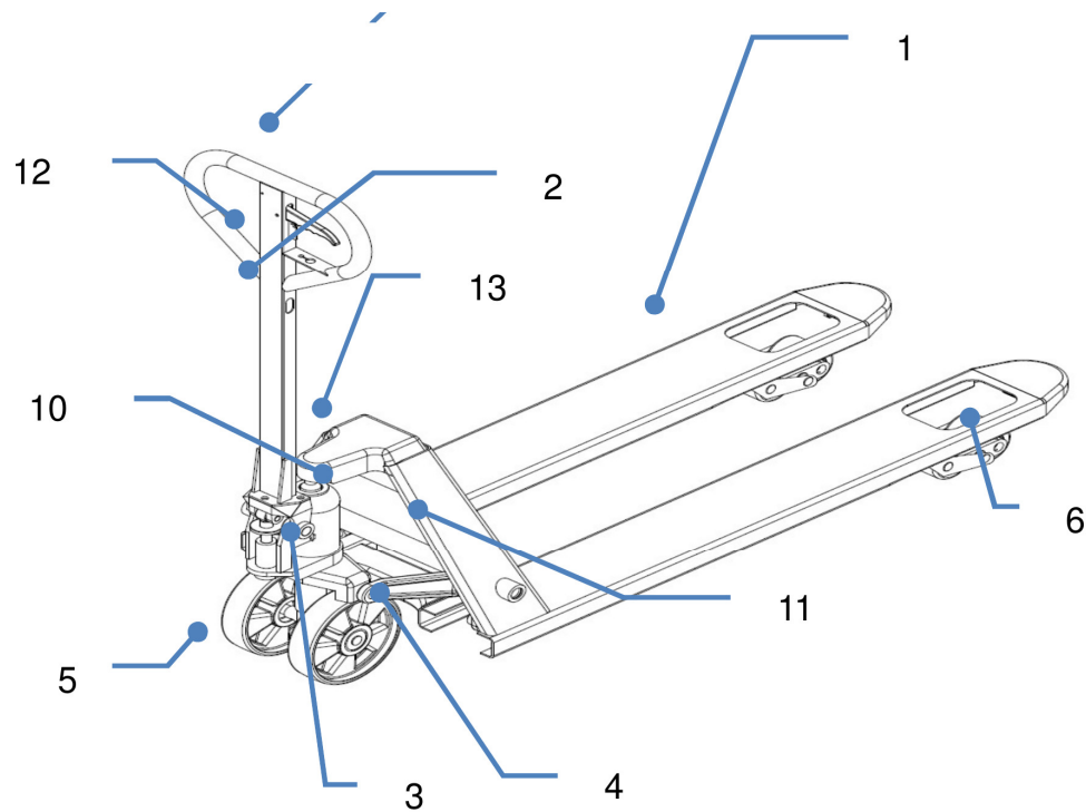
FIG. 2 — Componentes principais
