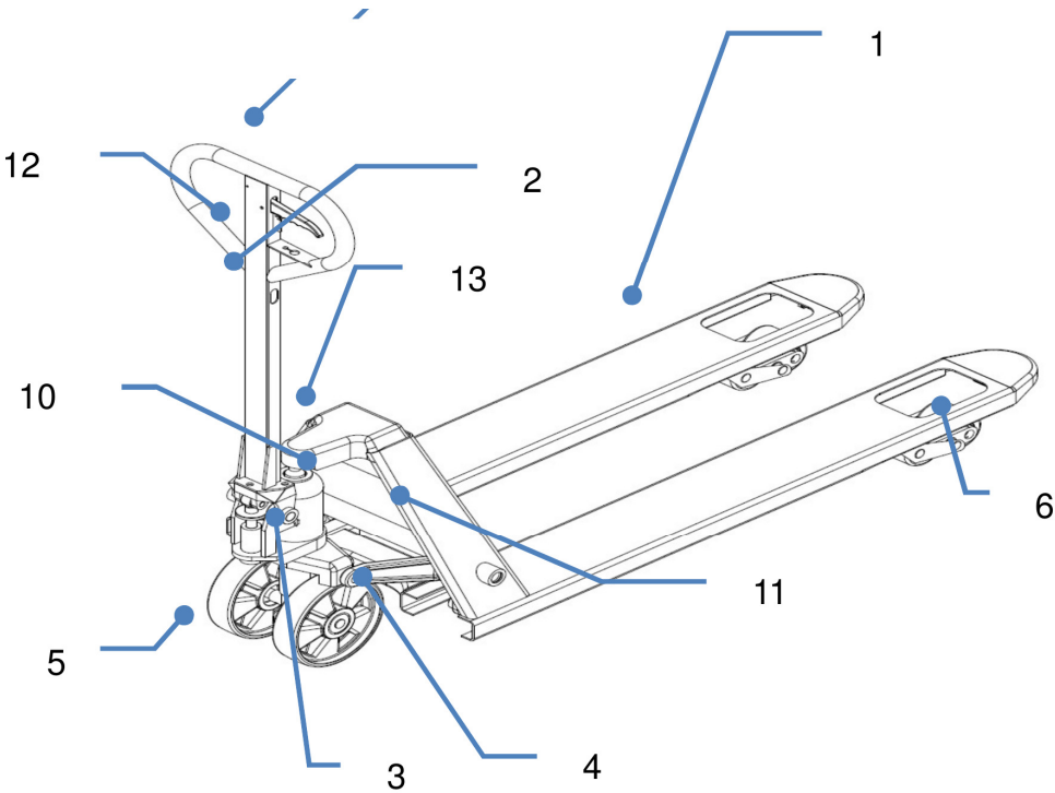
FIG. 2 — Componentes principais
