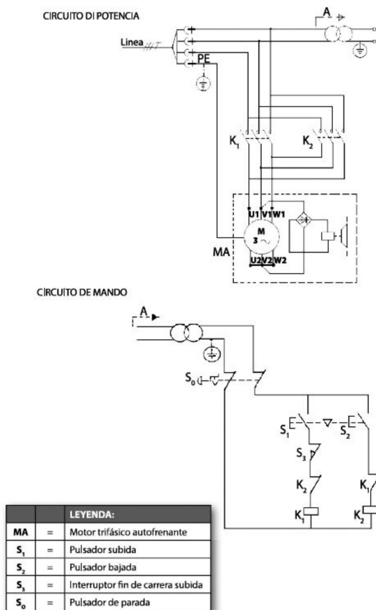
FIG. 18 — Esquema elétrico trifásico com telecomando de 2 teclas
