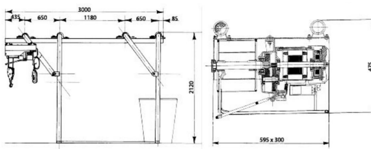
FIG. 1 — Dimensões gerais com suporte de cavalete
