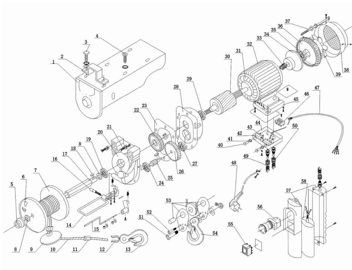
Vista explodida do elevador elétrico de cabo
