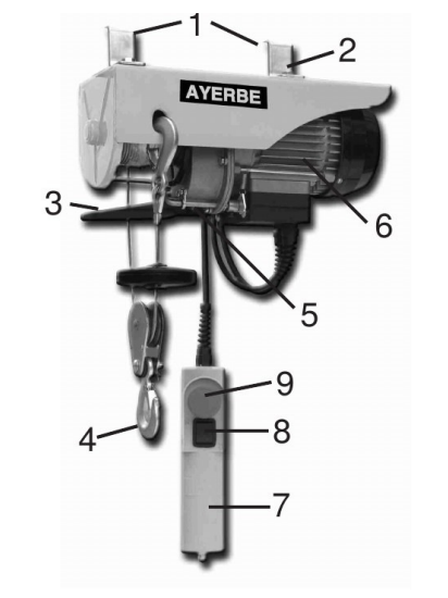
FIG. 1 — Elevador elétrico de cabo e componentes
