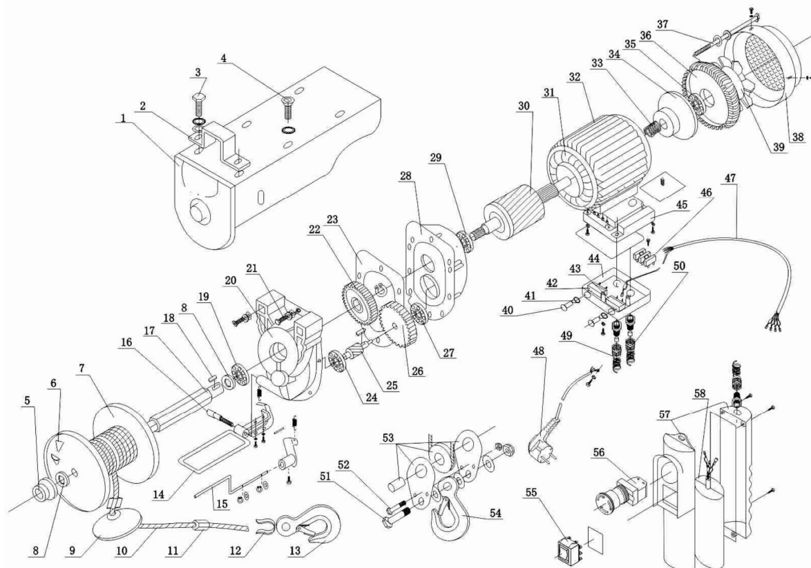
Vista explodida do elevador elétrico de cabo
