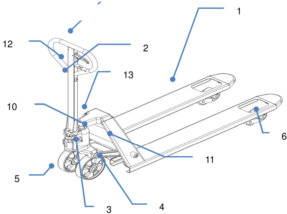
FIG. 2 — Componentes principais
