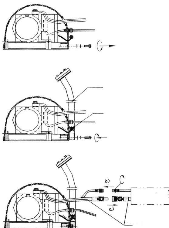
FIG. 3 — Sequência de montagem e ligação do grupo hidráulico.
