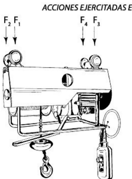
FIG. 2 — Actions exercées sur les galets de roulement
