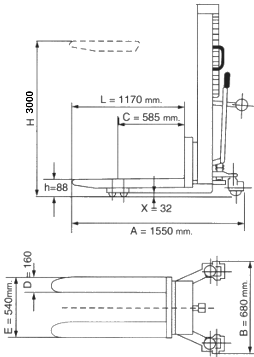
FIG. 1 — Dimensions principales
