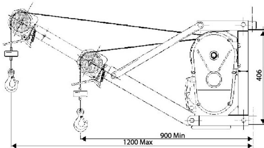
FIG. 1 — Dimensions générales de l'élévateur
