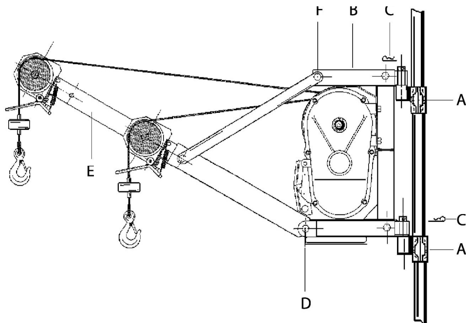
FIG. 3 — Installation de l'élévateur sur étau ou structure porteuse
