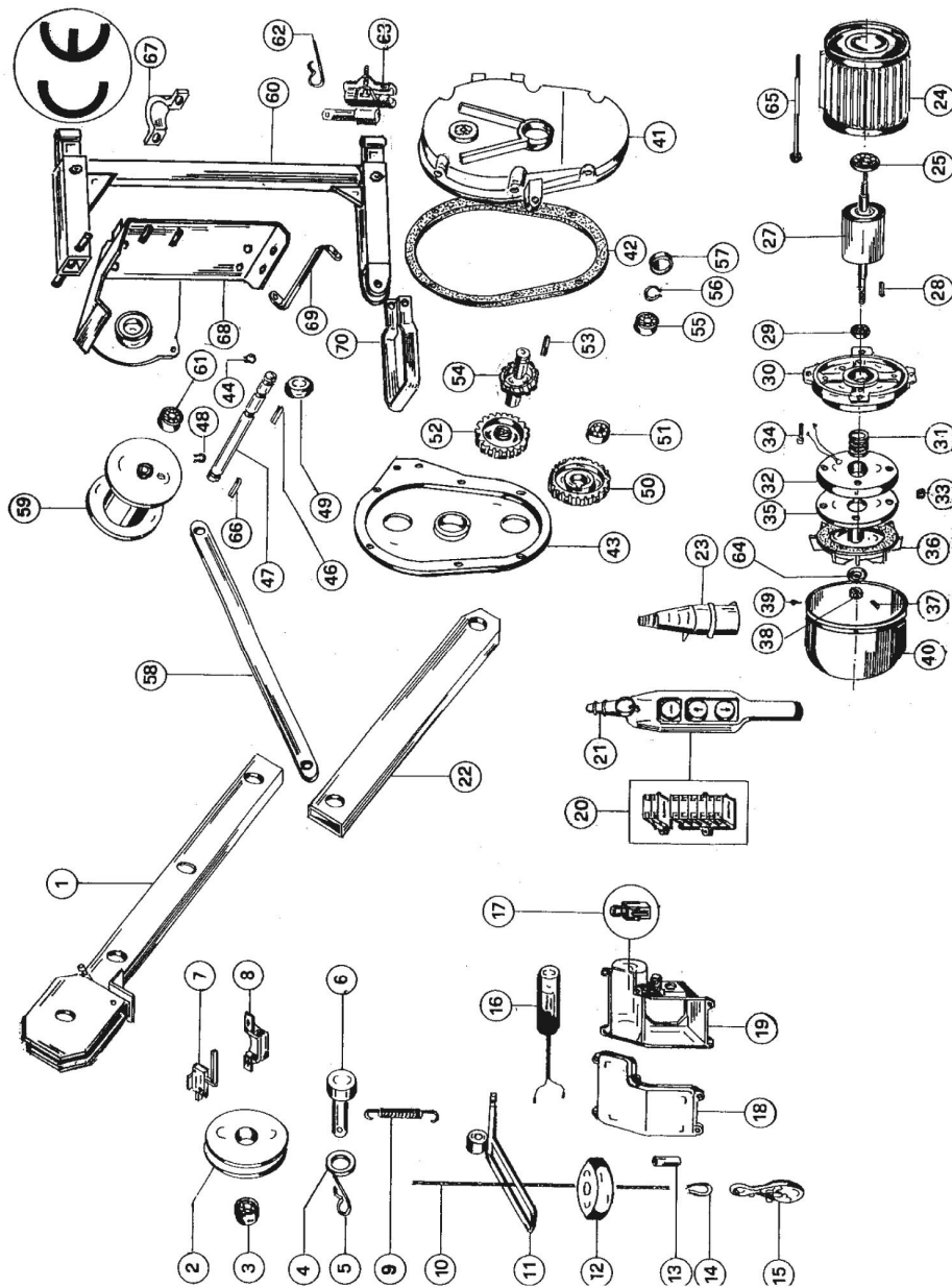
FIG. 12 — Vue éclatée AY-200 GR
