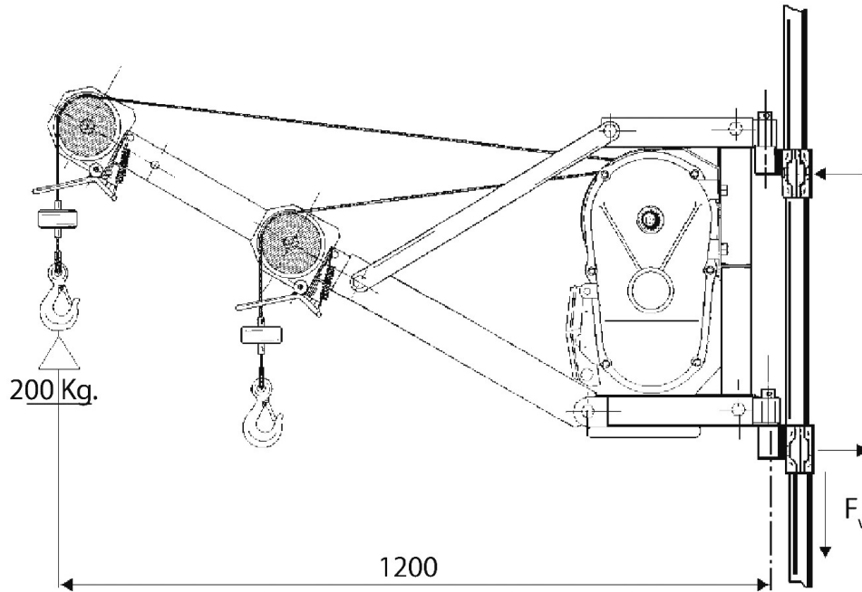
FIG. 4 — Forces exercées sur la structure
