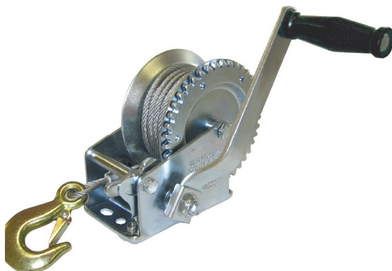
FIG. 1 — Treuil manuel AY-550-HW (réf. 585000).
