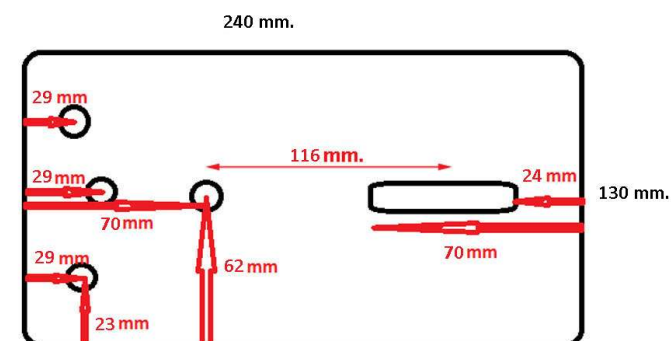
PLACA BASE CABRESTANTE MANUAL AY 1200
