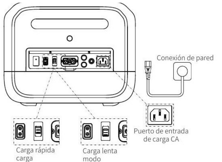
FIG. 4 — Carga desde la red eléctrica y selección de la velocidad de carga
