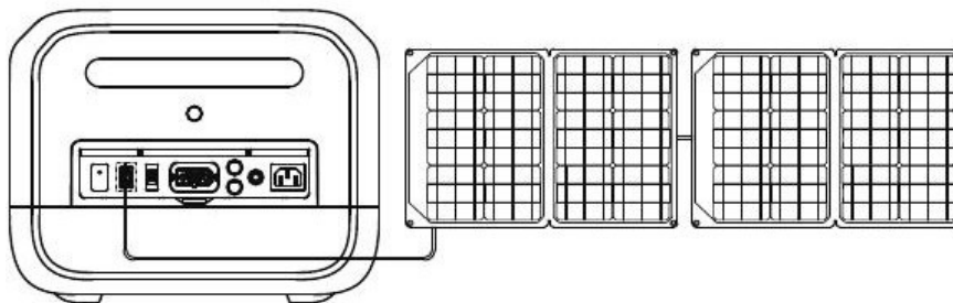
FIG. 7 — Carga con dos paneles solares conectados en serie
