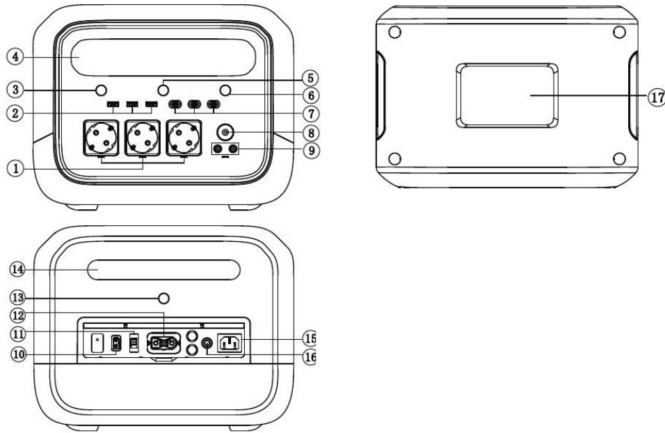
FIG. 2 — Componentes principales: frontal, cara superior y cara posterior
