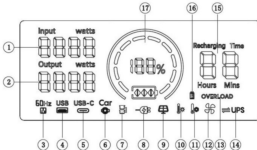
FIG. 3 — Indicaciones de la pantalla LCD
