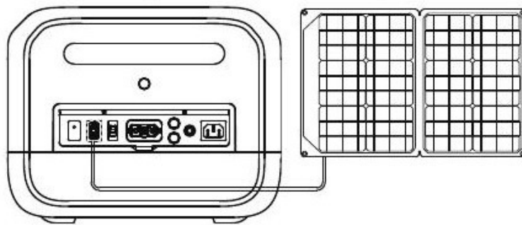
FIG. 6 — Carga con un panel solar
