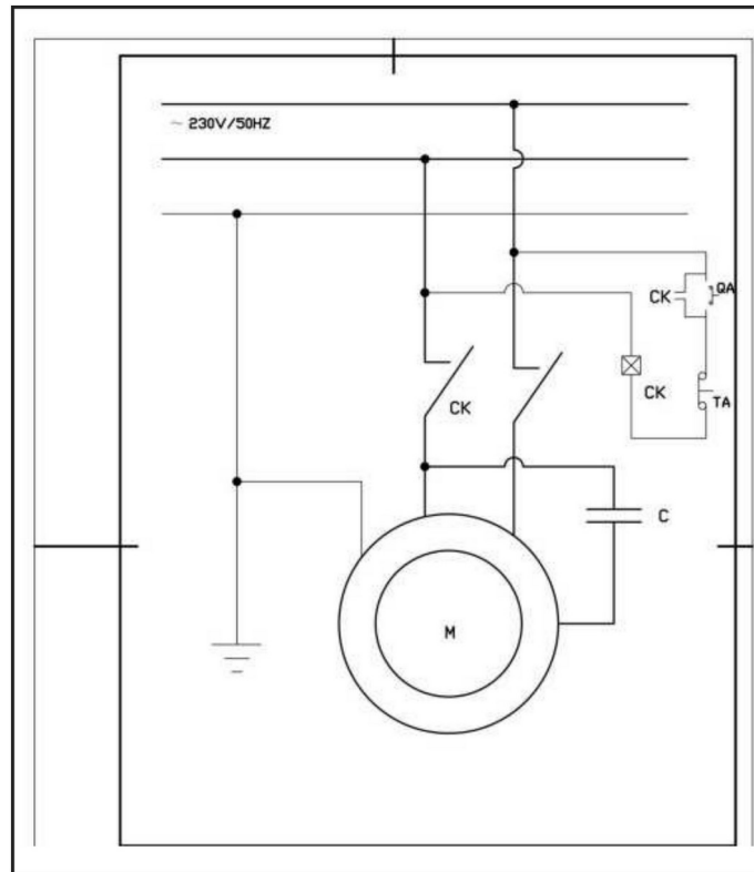
FIG. 5 — Esquema de conexiones
