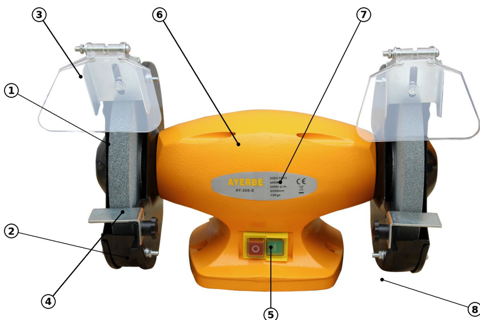
FIG. 1 — Componentes (AY-200 E; la AY-150 E es idéntica salvo el tamaño de la muela)
