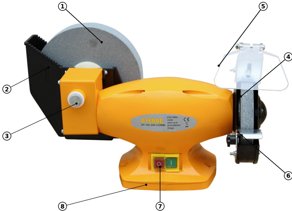
FIG. 2 — Componentes de la AY-150-200 COMBI
