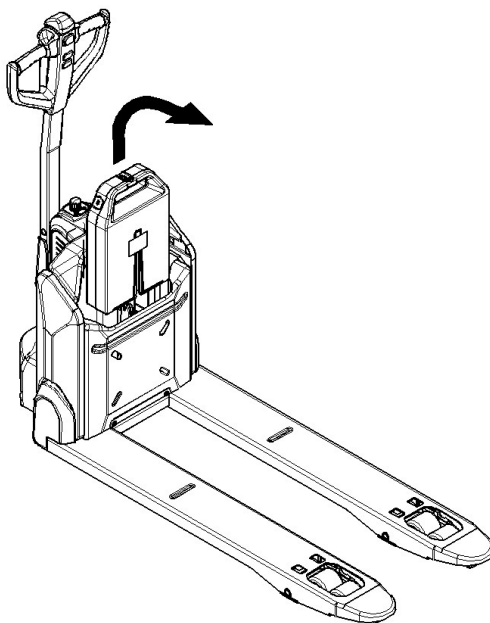
FIG. 13 — Extracción e instalación de la batería.
