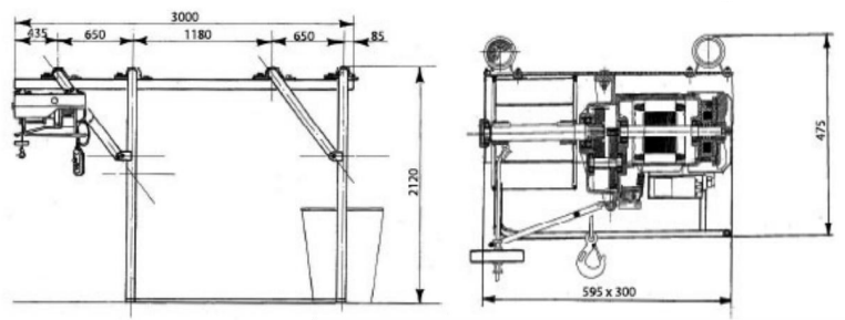
FIG. 1 — Dimensiones generales con soporte a caballete
