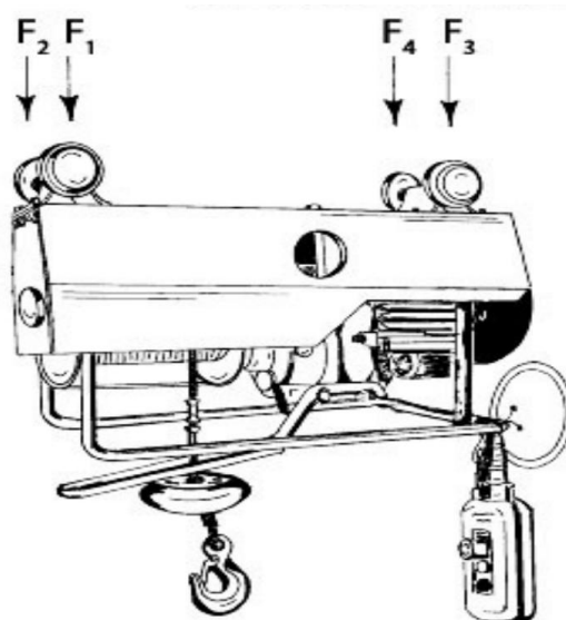
FIG. 2 — Acciones ejercidas en las ruedas de deslizamiento
