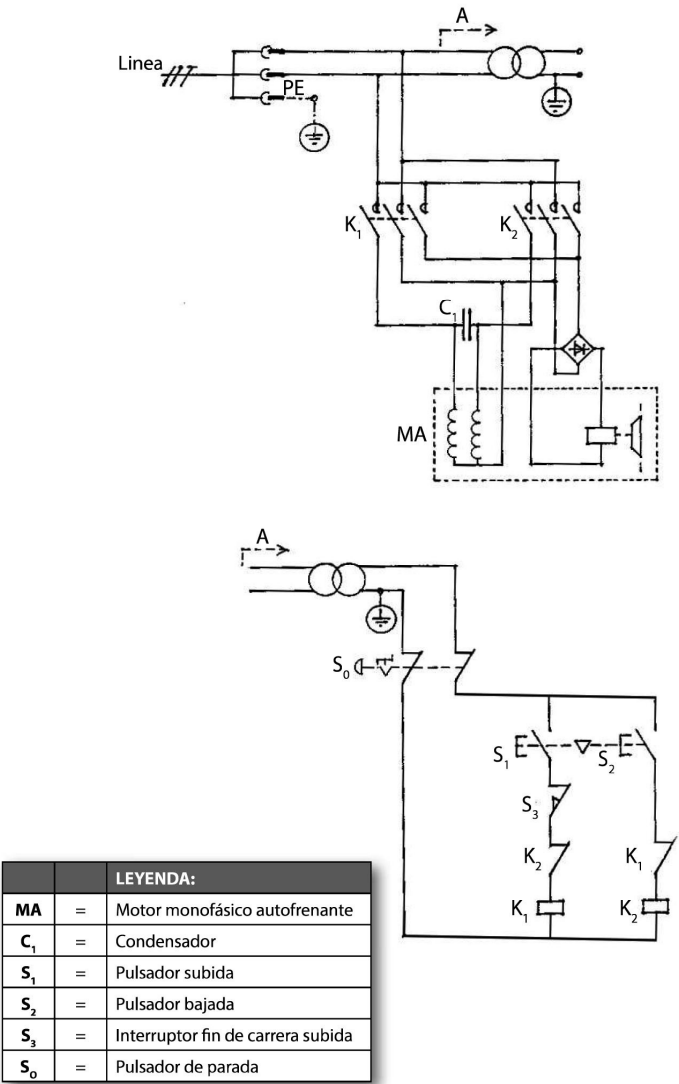
FIG. 13 — Esquema eléctrico
