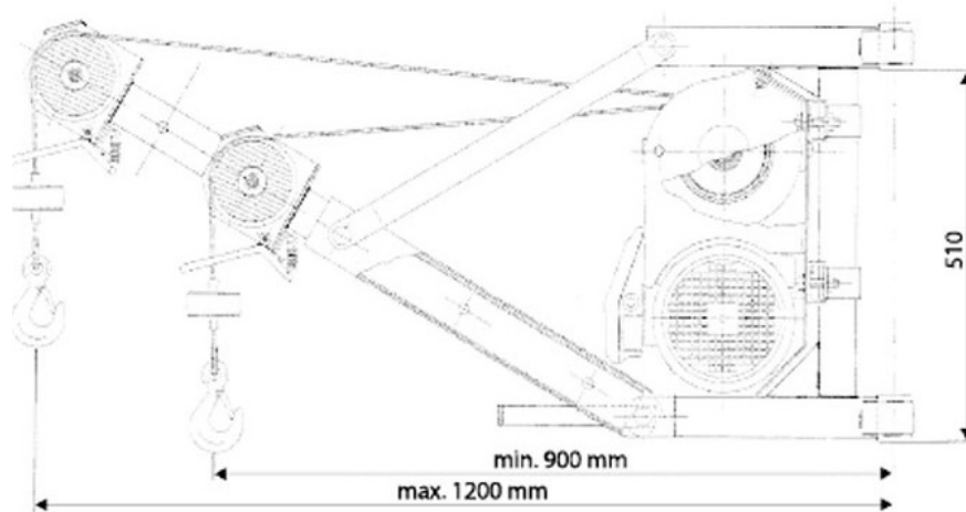
FIG. 1 — Dimensiones generales del elevador
