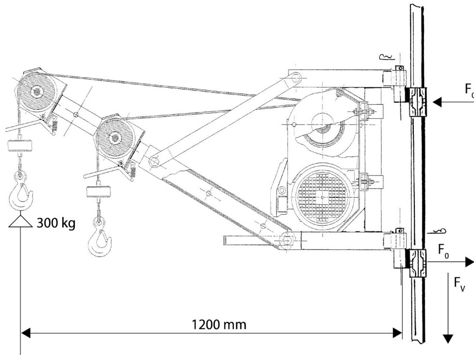
FIG. 4 — Fuerzas ejercidas sobre la estructura
