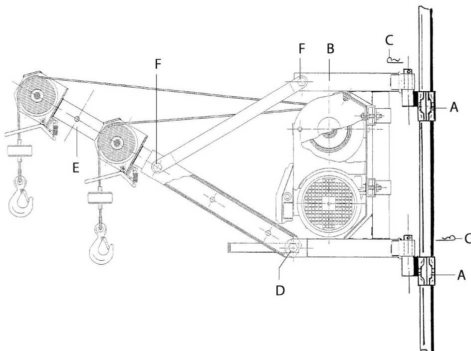
FIG. 3 — Instalación del elevador sobre puntal o estructura portante
