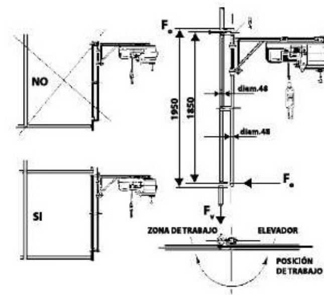
FIG. 3 — Unión a andamiaje
