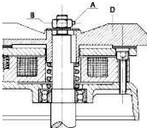
FIG. 9 — Reglaje del freno
