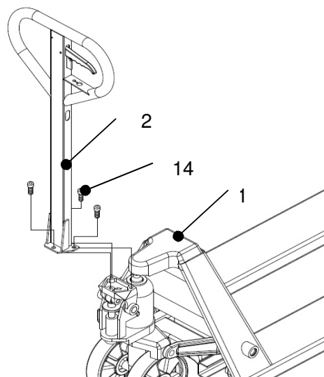
Fig.8 Ensamblaje del mango.
