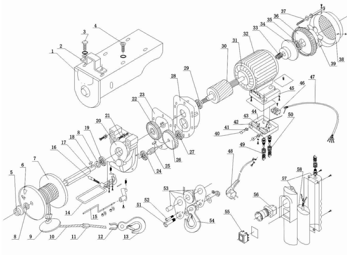
Despiece del elevador eléctrico de cable
