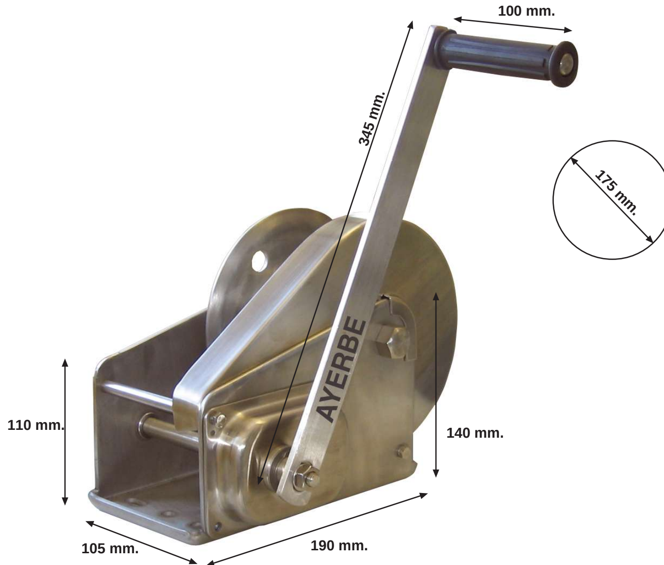
PLACA BASE CABRESTANTE MANUAL AY 800
