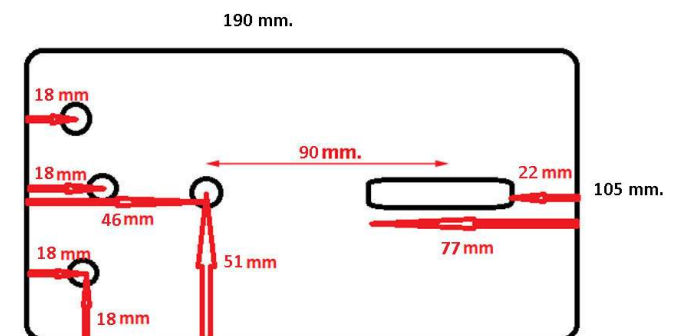
PLACA BASE CABRESTANTE MANUAL AY 800
